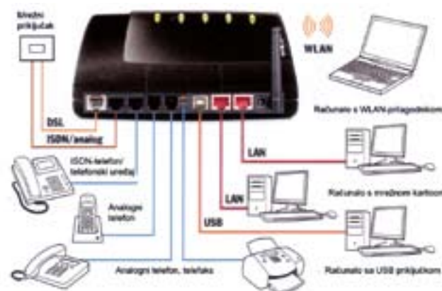
Usmjernik (router) s brojnim mogućnostima
