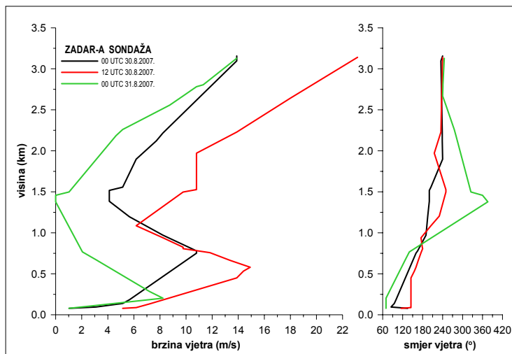
Vertikalni profili brzine i smjera vjeta za Zadar-aerodrom do 3 km visine prema radiosondažnim podacima za 30. kolovoza 2007.
